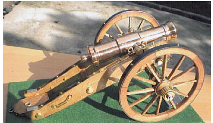
Bombavető tarack részcsővel (7 fontos réz) M: 1:10
